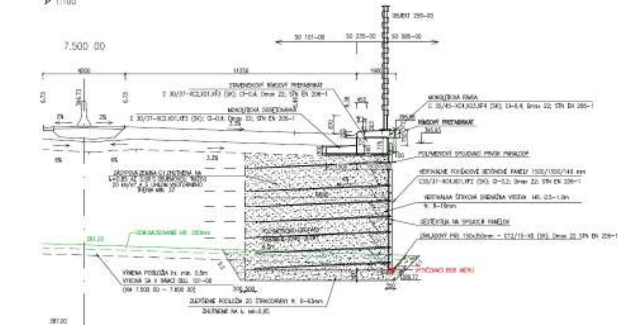
Vzorový priečný rez
