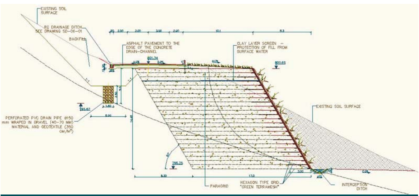
Поперечное сечение
