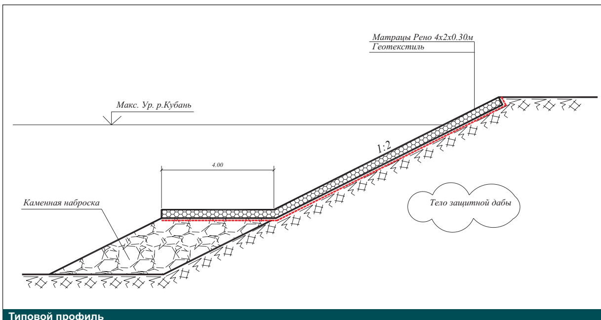
Типовой профиль
