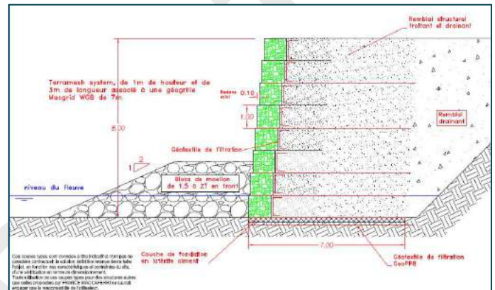
Figure 1 : coupe type du projet
