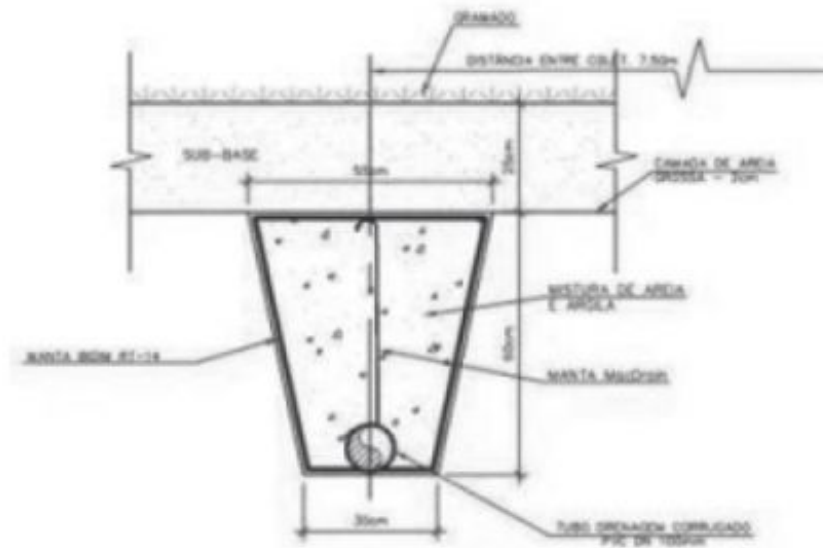
6 DETALHE DO DRENOS TRANSVERSAIS ALTERNATIVA - 1 ESCALA 1:20
